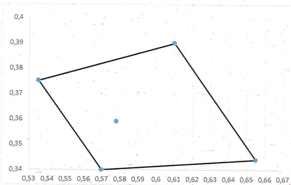
Допустимая область для оранжевого флуоресцентного цвета и фактические координаты цветности образца (брюки)
